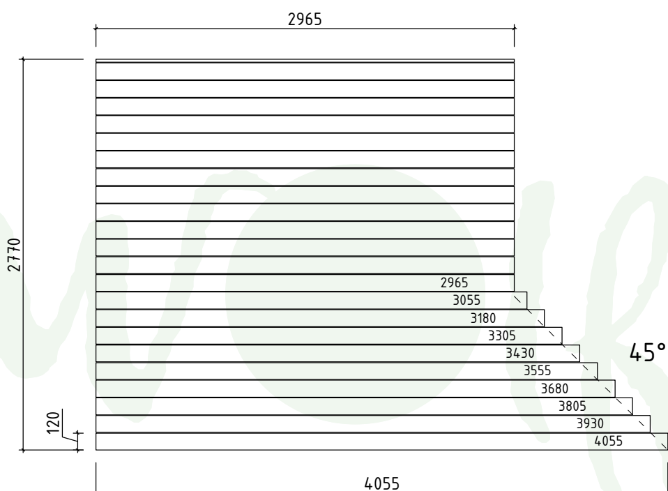
Terrassenbretter 120x28
