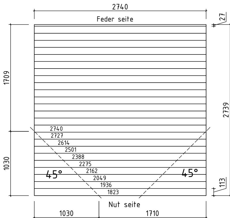
Terrassenbretter 120x28
