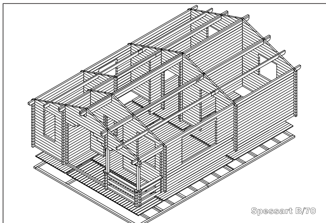
3D-Ansichtsplan
